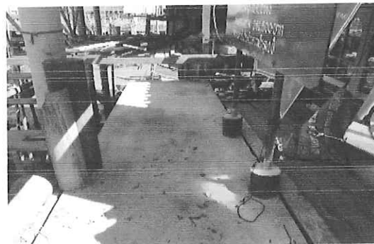
๔๒.โครงการก่อสร้างสะพานเดินเท้า คสล.สายบ้านนายบุญมี - นายมิตร หมู่ที่ ๒
